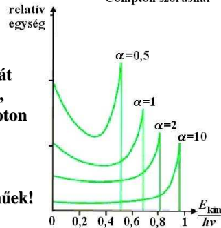
A meglökött elektronok energiaeloszlása Compton szórásnál
